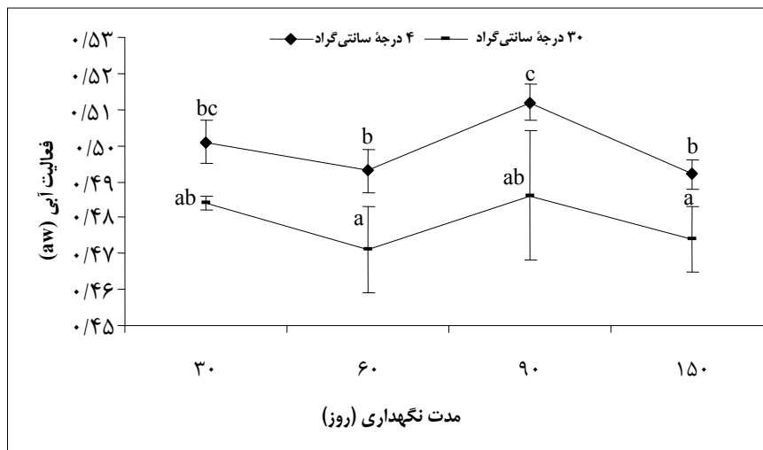
شکل ۵- مقایسه میانگین اثر دما و مدت نگهداری بر فعالیت آبی خرماهای سایر پس از ۳۰، ۶۰، ۹۰ و ۱۵۰ روز نگهداری
