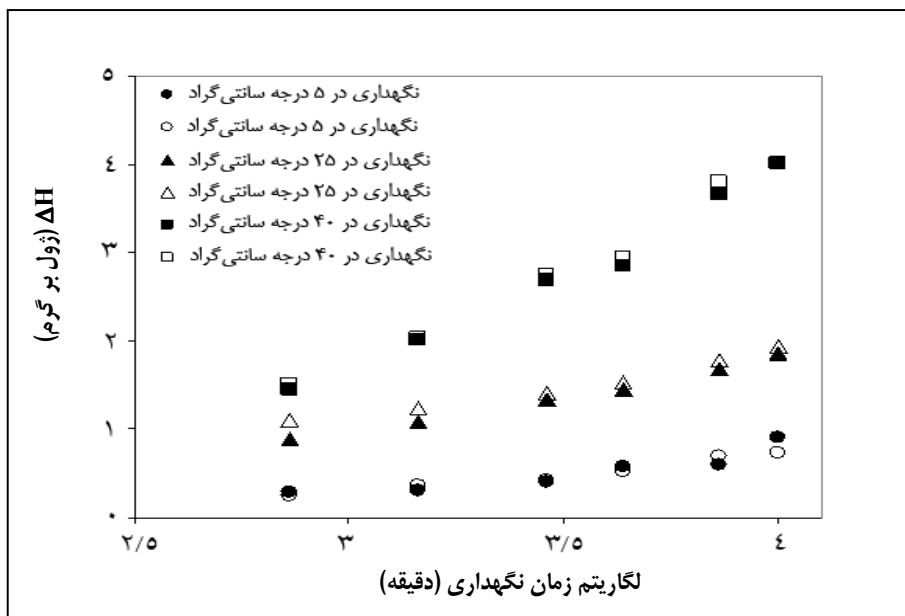
شکل ۶- اثر دمای نگهداری بر سینتیک تغییر انتالپی در نمونه PCGP ژلاتین با ۱۱ درصد رطوبت (بر اساس وزن تر). اندازه‌گیری‌ها در ۲ تکرار با نشانه‌های پر و توخالی نشان داده شده‌اند.
