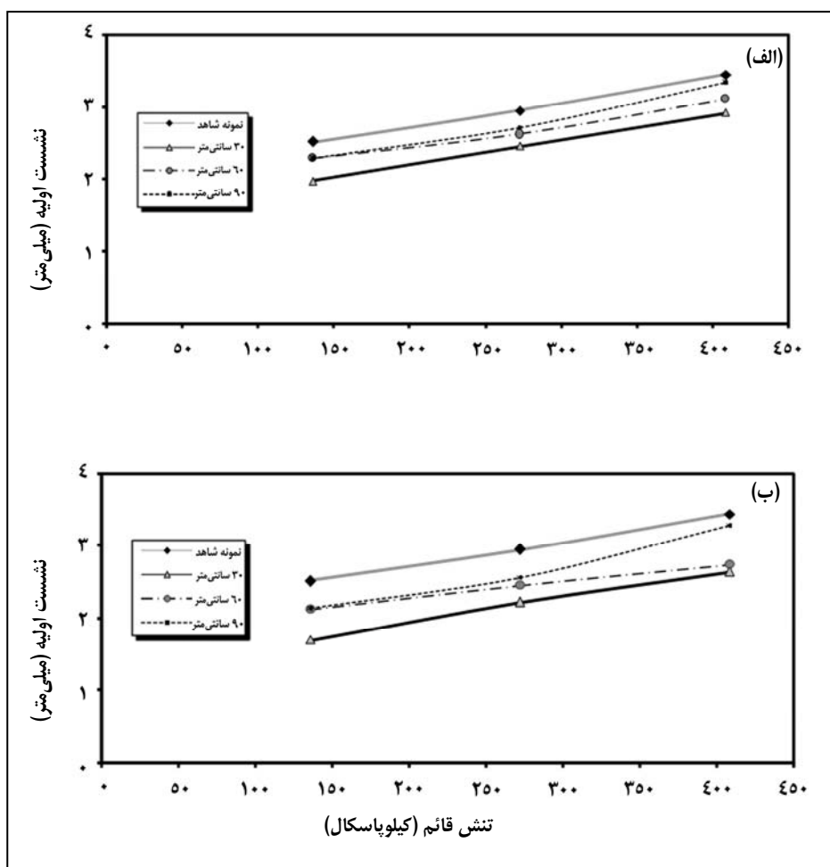
شکل ۶- تأثیر فاصله از منبع تغذیه بر نشست اولیه نمونه‌ها در دستگاه برش مستقیم؛ (الف) نمونه ۲۰ روز؛ و (ب) نمونه ۴۰ روز
